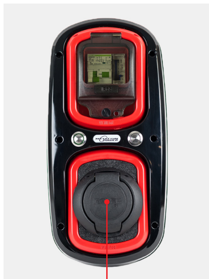
7KW SOCKET
